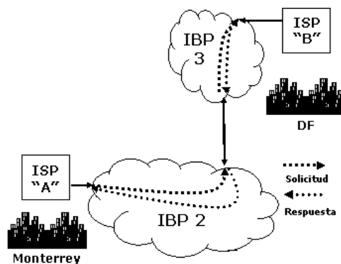
Figura 9: Un IBP de menor tamaño, tomando de ventaja de un acuerdo de interconexión con un IBP con una red más grande.
